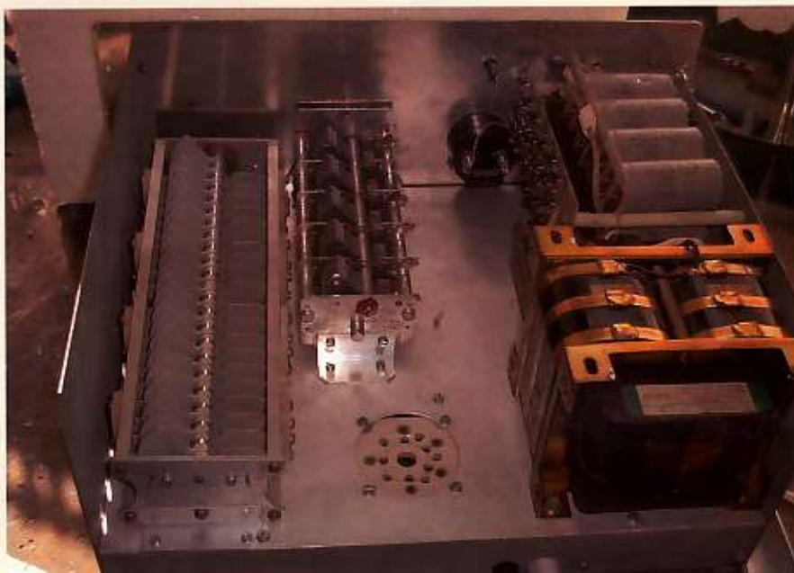
Foto 1: Opstelling van de beide afstemcondensatoren.
